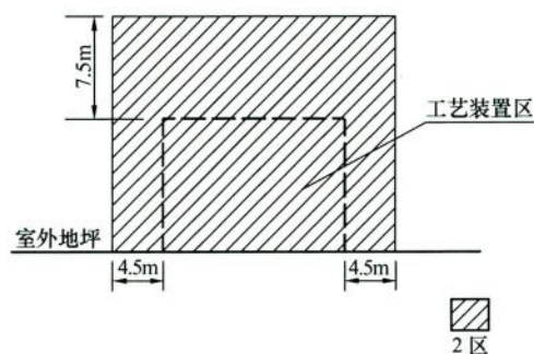
图 D-5 露天设置的工艺装置区的爆炸危险区域等级和范围划分
