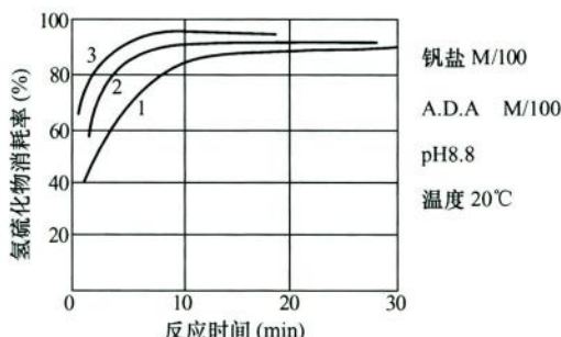
图 1 不同硫容量和反应时间消耗氢硫化物的百分比图
